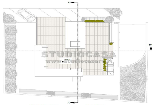
PIANTA COPERTURA scala 1:100 Attiva Windows Prese e Impostazioni per attivare Win
